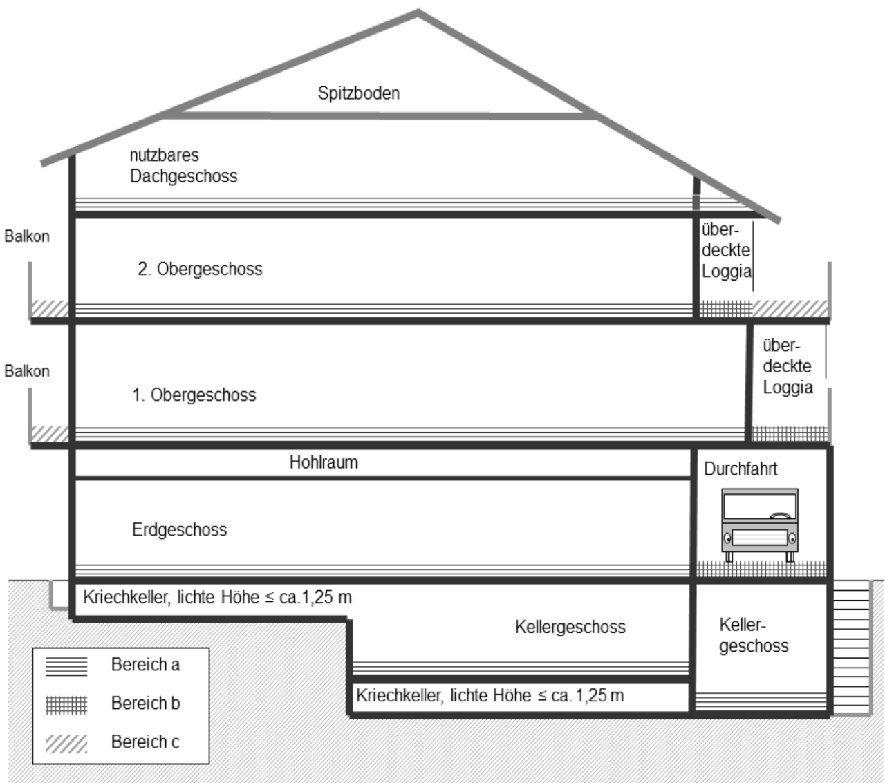
Abbildung: Zuordnung der Grundflächen zu den Bereichen a, b und c
